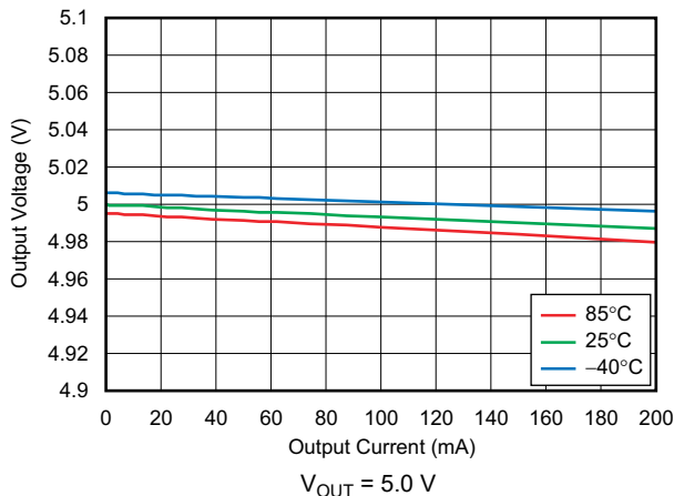
图 6-3. Load Regulation
