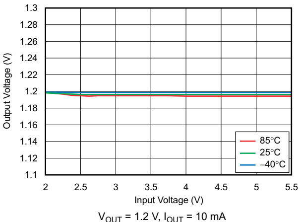
图 6-4. Line Regulation
