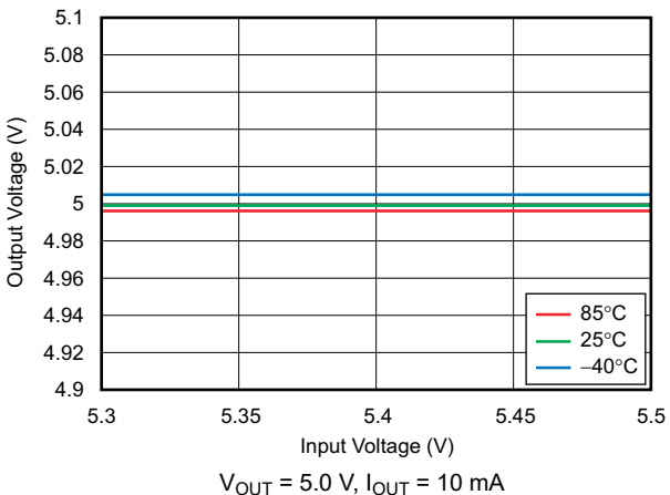
图 6-6. Line Regulation
