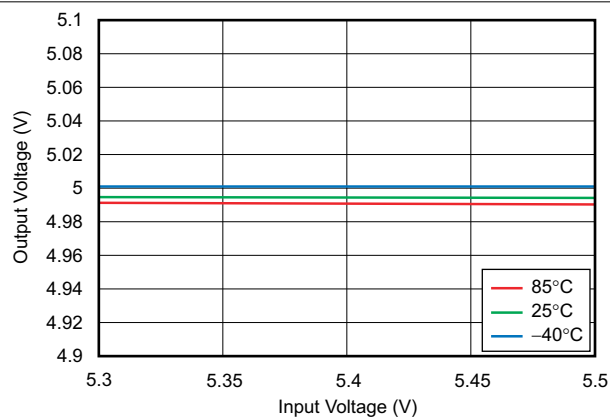
图 6-7. Line Regulation
