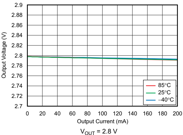
图 6-2. Load Regulation
