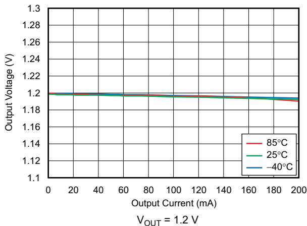
图 6-1. Load Regulation
