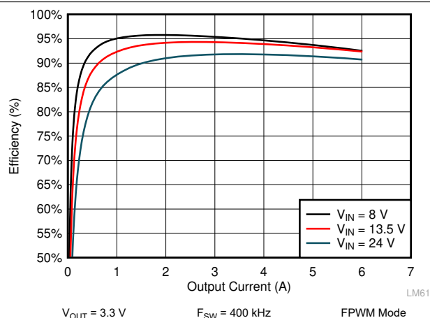
图 10-6. LM61460-Q1 Efficiency
