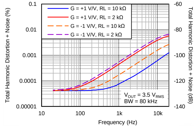
图 26. THD+N 比与频率间的关系
