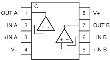
D 和 DGK 封装 : OPA2192 8 引脚 SOIC 和 VSSOP 俯视图
