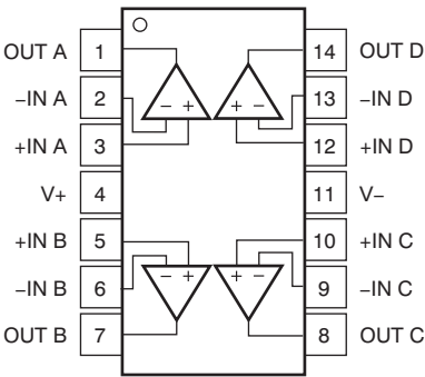
D 和 PW 封装 : OPA4192 14 引脚 SOIC 和 TSSOP 俯视图
