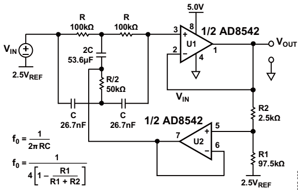
图36. 60Hz双T陷波滤波器，Q = 10
