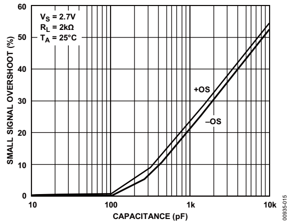
图15. 小信号过冲与负载电容的关系
