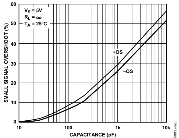
图27. 小信号过冲与负载电容的关系
