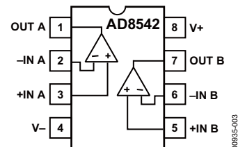
图3. 8引脚SOIC封装、8引脚MSOP封装和8引脚TSSOP封装 (R、RM和RU后缀)
