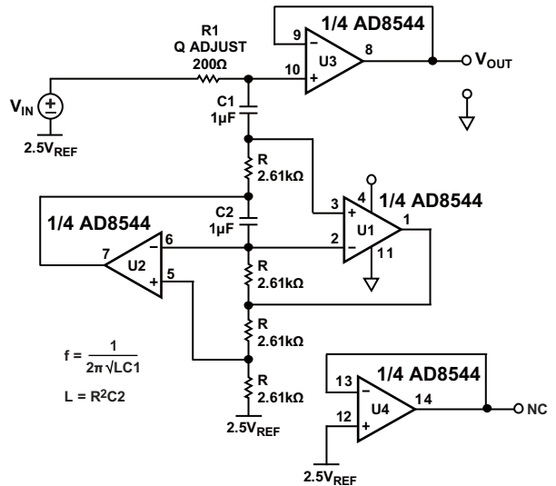
图38. 具有输出缓冲器的FDNR 60 Hz陷波滤波器
