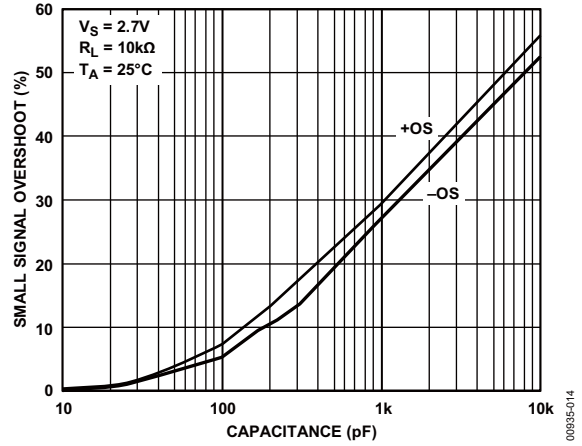
图14. 小信号过冲与负载电容的关系
