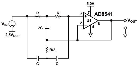
图37. 60Hz双T陷波滤波器，Q = ∞ (理想情况)
