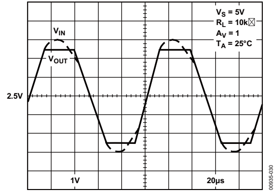
图31. 无倒相
