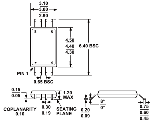
图46. 8引脚超薄紧缩小型封装[TSSOP] (RU-8)
