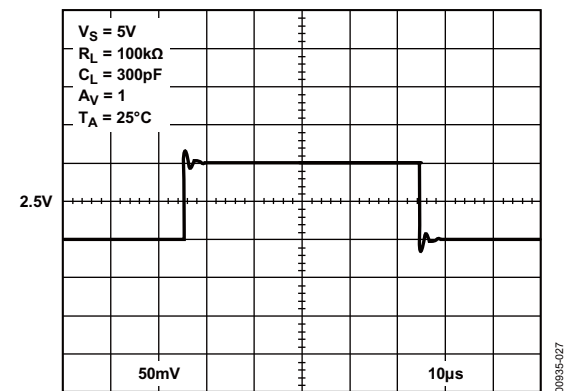
图28. 小信号瞬态响应
