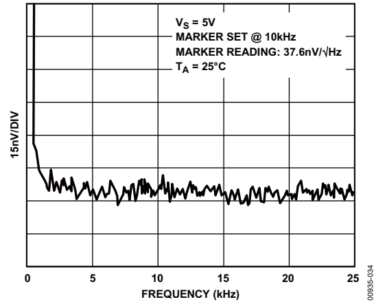
图35. 电压噪声
