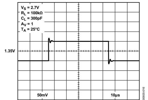
图16. 小信号瞬态响应
