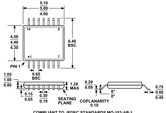
图42. 14引脚超薄紧缩小型封装[TSSOP] (RU-14)
