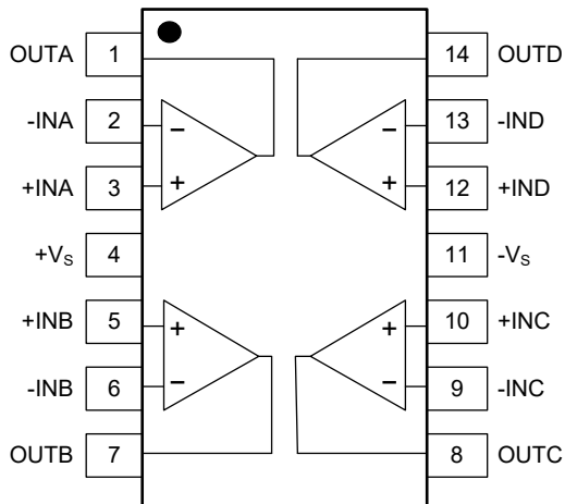
SOIC-14
