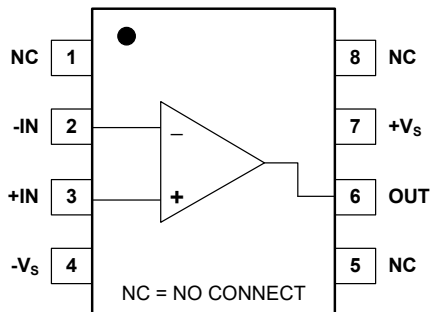
SOIC-8/MSOP-8
