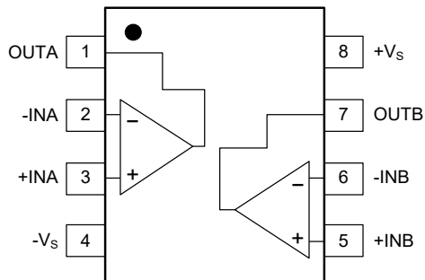
SOIC-8
