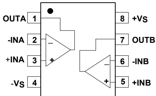
SOIC-8
