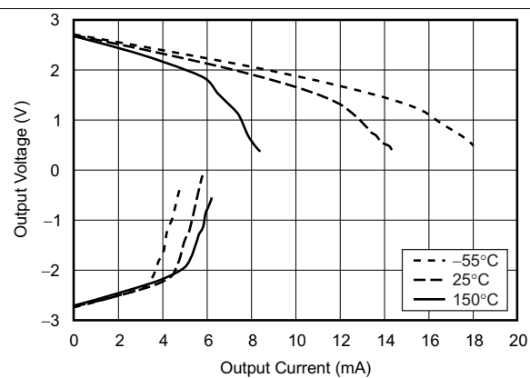
图 12. 输出电压摆幅与输出电流间的关系
