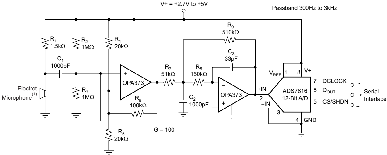
图 30. OPA2373 作为语音旁滤波的数据采集系统
