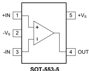
SOT-553-5
