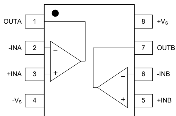
SOIC-8
