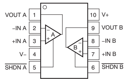
OPA2320S DGS 封装 10 引脚 VSSOP 俯视图
