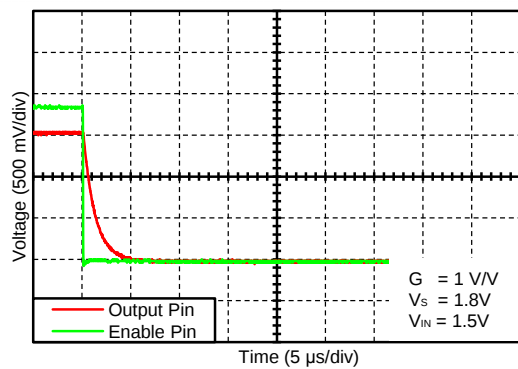
图 31. 启用关断
