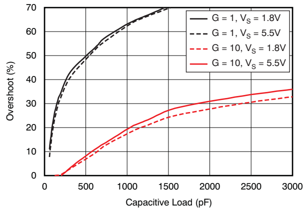
图 37. 小信号过冲与容性负载间的关系 ( 100\text{mV}_{\text{pp}} 输出阶跃)
