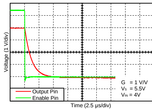
图 32. 启用关断
