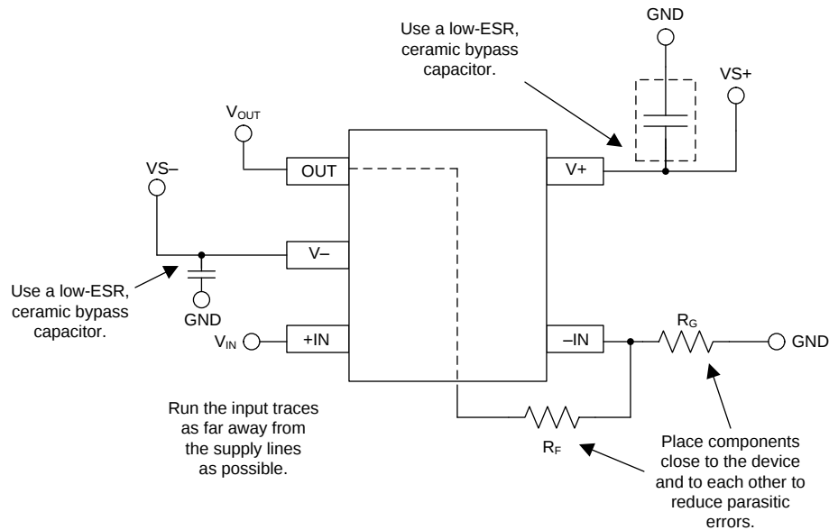
图 49. 布局示例
