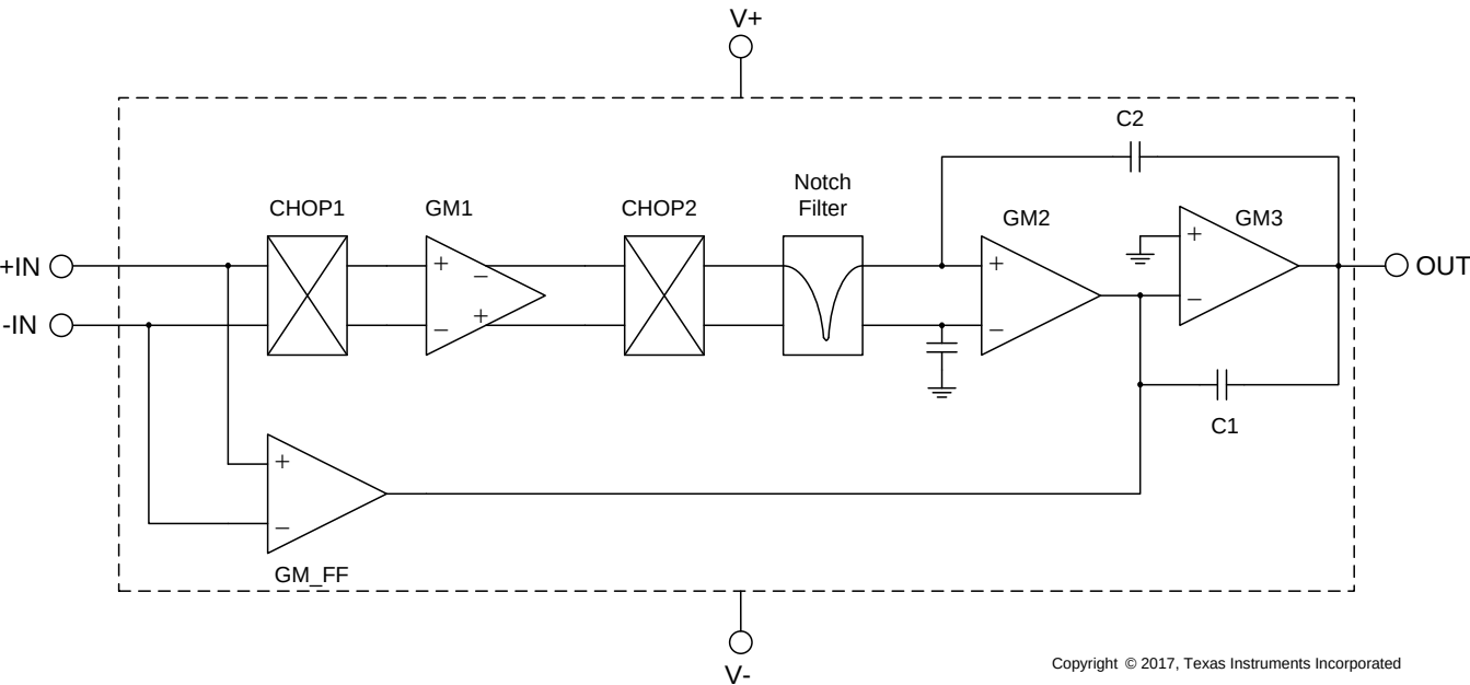
图 38. 功能框图
