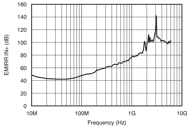
图 40. EMIRR 测试
