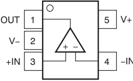
OPA188 DBV 封装 5 引脚 SOT-23 俯视图
