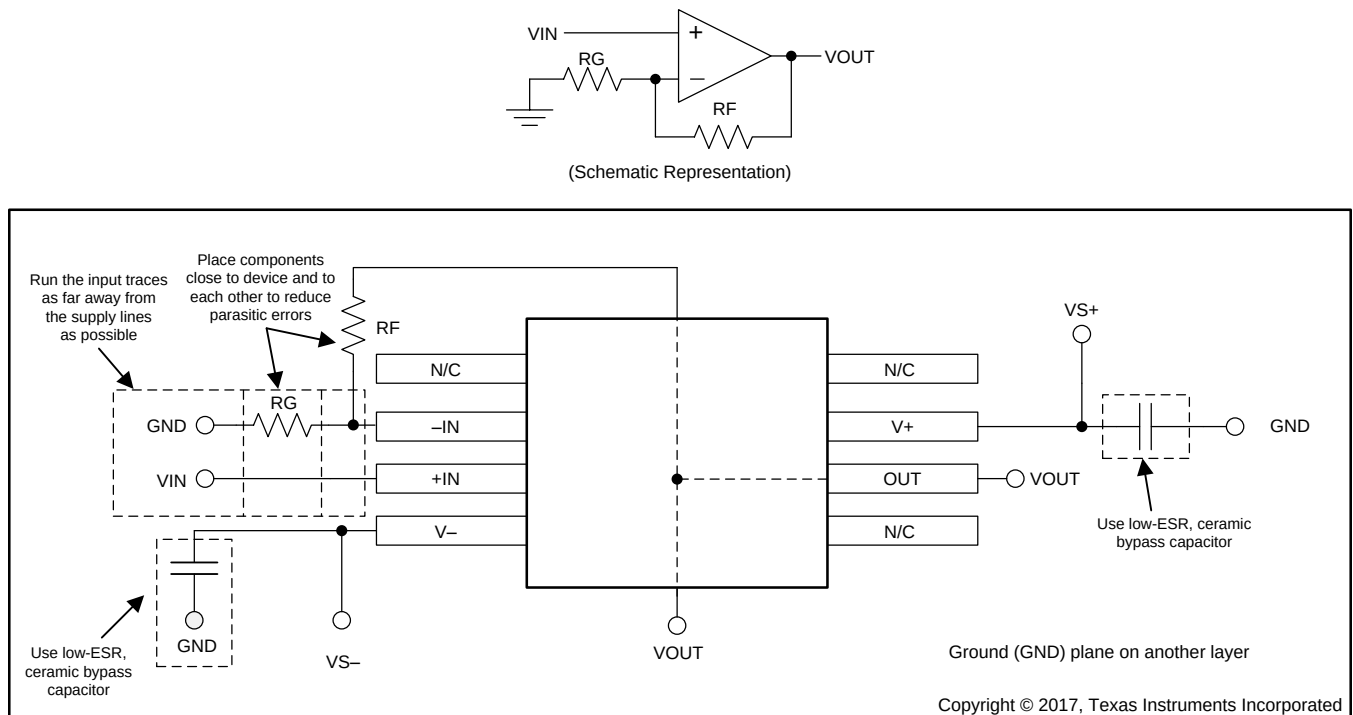
图 51. 布局示例
