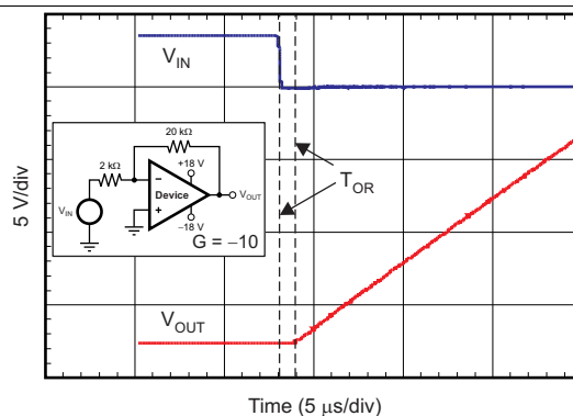
图 26. 无相位反转
