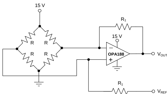
图 47. 桥式放大器
