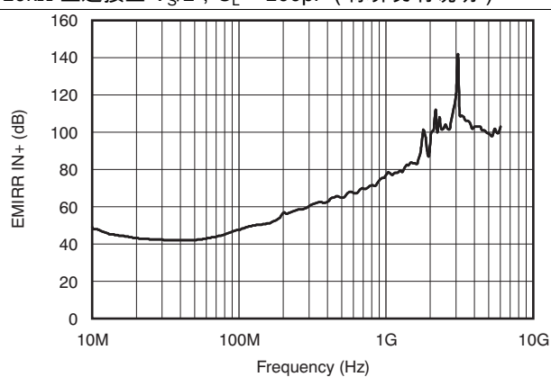
图 37. EMIRR IN+ 与频率间的关系
