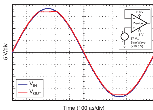
图 39. 无相位反转
