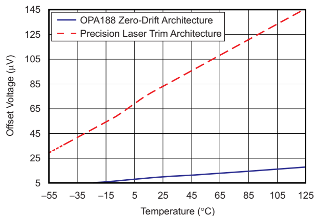
采用自动归零技术实现超低温度漂移
