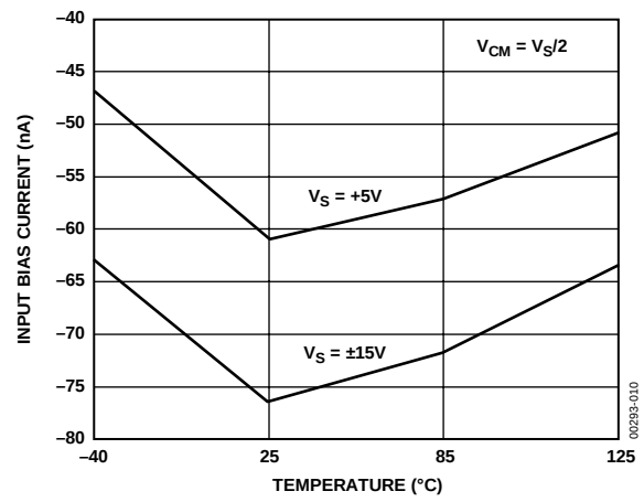
图10. 偏置电流与温度的关系
