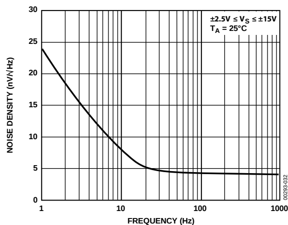
图32. 电压噪声密度与频率的关系
