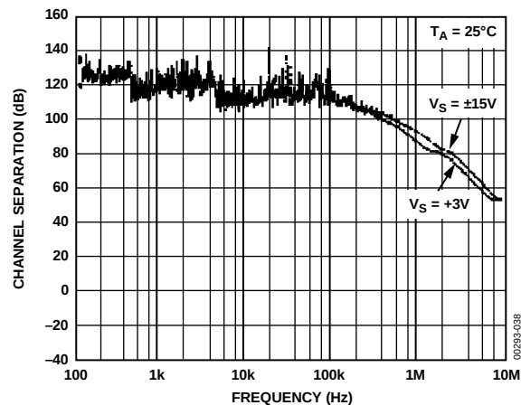
图38. 通道隔离与频率的关系
