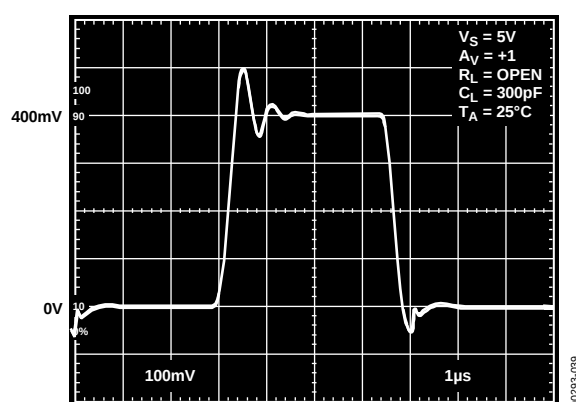
图39. 小信号瞬态响应
