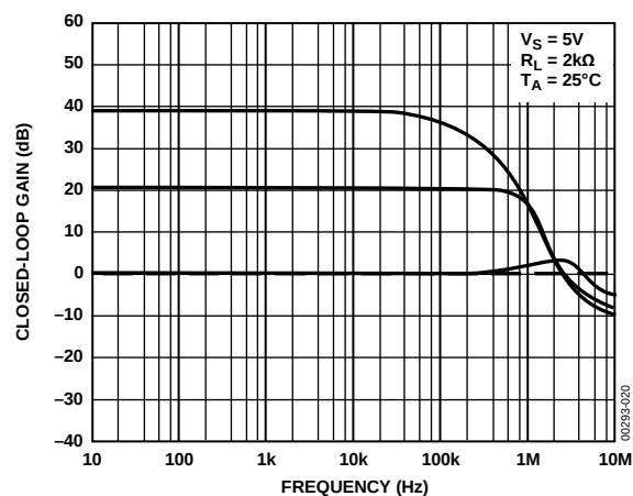
图20. 闭环增益与频率的关系(2 kΩ负载)
