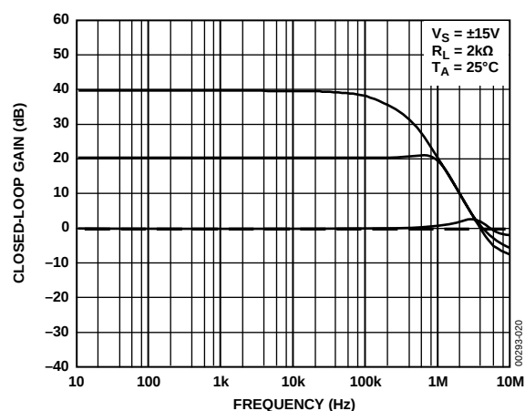
图21. 闭环增益与频率的关系(2 kΩ负载)
