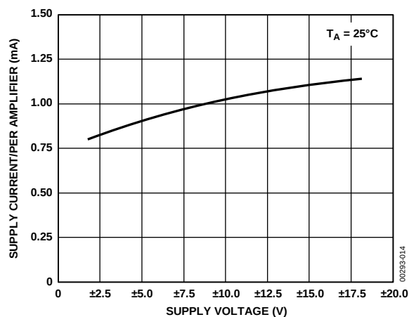
图14. 电源电流与电源电压的关系
