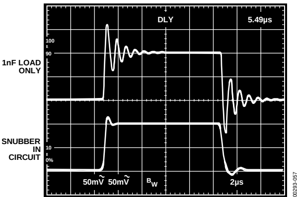
图57. 增加一个缓冲器网络与1 nF负载并联可降低过冲和响铃振荡
