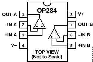
图2. 8引脚PDIP(P后缀)和8引脚SOIC(S后缀)
