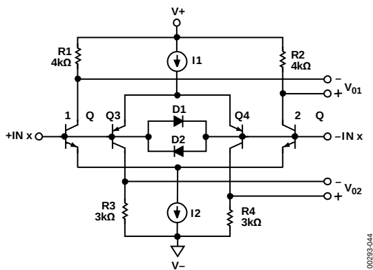
图44. OP284等效输入电路
