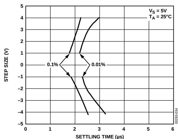
图34. 阶跃大小与建立时间的关系
