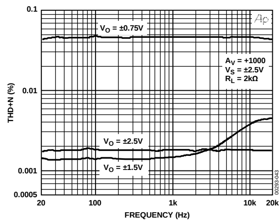
图43. 总谐波失真加噪声与频率的关系
