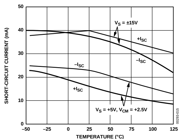
图15. 短路电流与温度的关系
