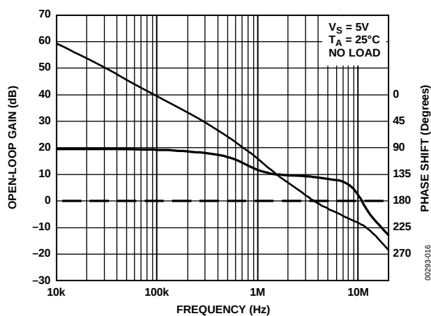
图16. 开环增益和相位与频率的关系(空载)
