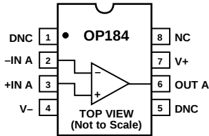
图1. 8引脚SOIC(S后缀)
