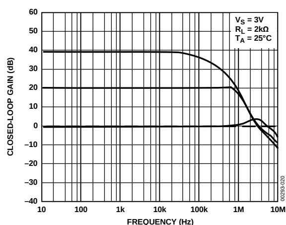
图22. 闭环增益与频率的关系(2 kΩ负载)
