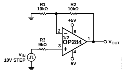
图51. 输出过载恢复时间的测试电路
