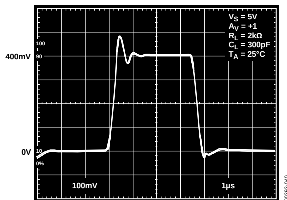
图40. 小信号瞬态响应
