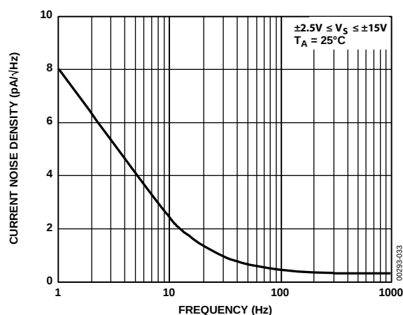
图33. 电流噪声密度与频率的关系
