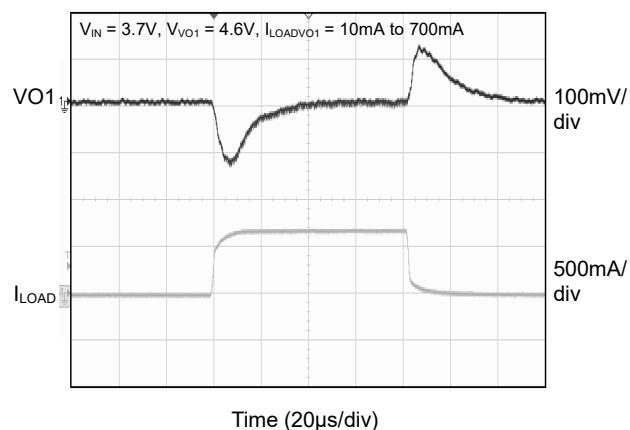
VO1 Load Transient
