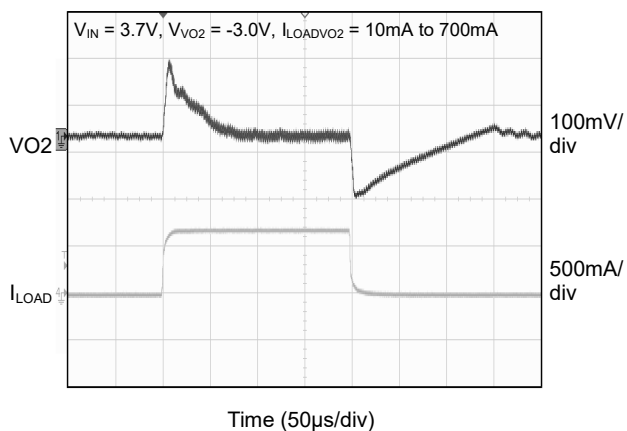
VO2 Load Transient
