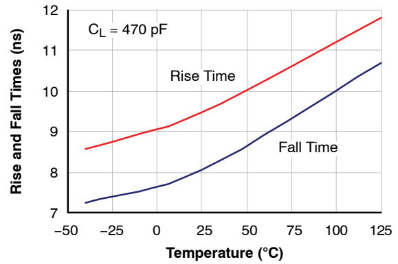
图 26. 上升和下降时间与温度的关系
