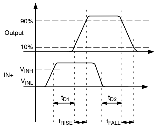
图 3. 非反向波形
