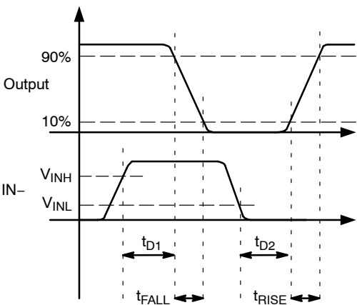
图 4. 反相波形
