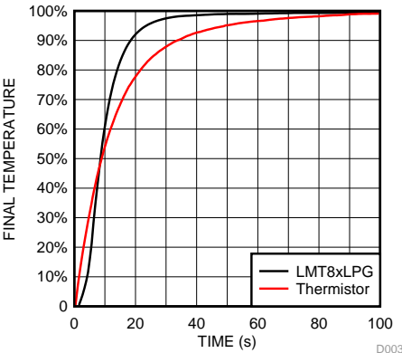
热时间常量
