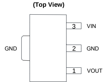
SOT89
