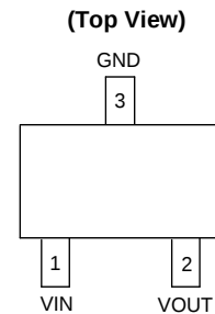
SOT23
