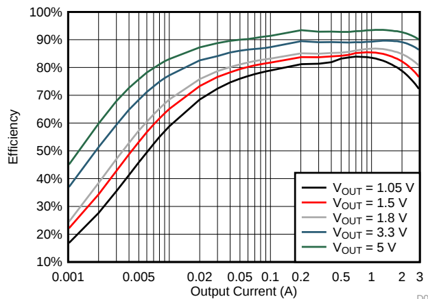
TPS563201 效率
