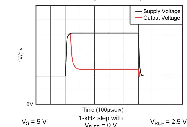
图 22. Brownout Recovery
