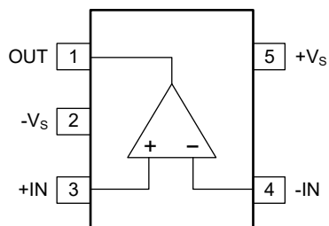
SC70-5/SOT-23-5
