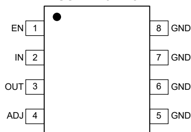
SOIC-8
