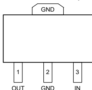
SOT-89-3
