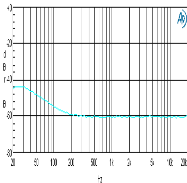
PSRR_F@12V 8OHM
