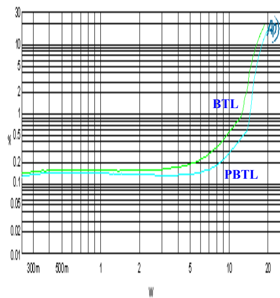
PBTTL@12V 4OHM
