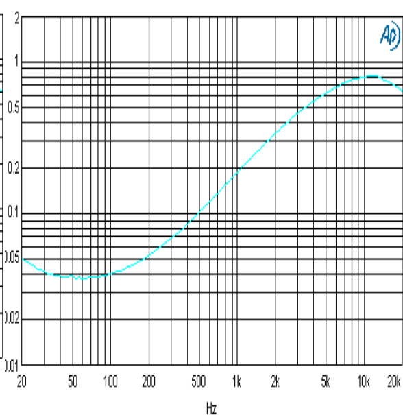
THDN_F@9V 4OHM 3W
