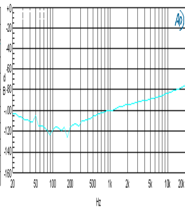
XTK_F@12V 8OHM
