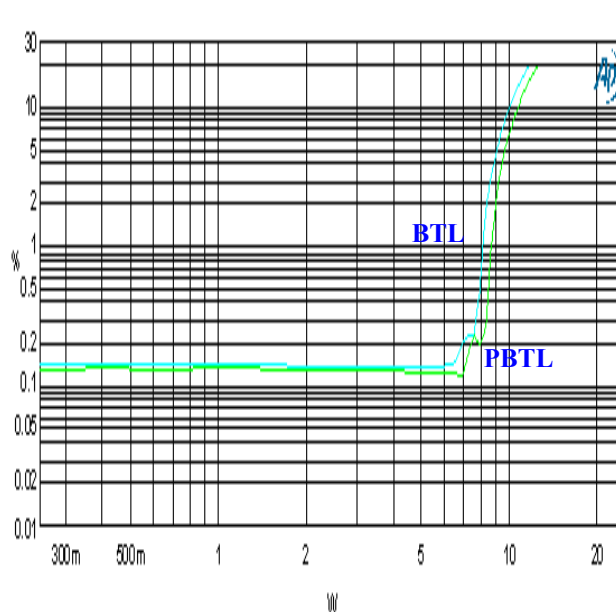
PBTTL@12V 8OHM
